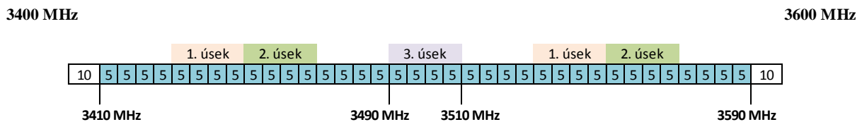
Obrázok 6.1: Návrh rozdelenia frekvenčného pásma 3400 – 3600 MHz na tri úseky, pričom každý úsek by mohol získať jeden podnik
