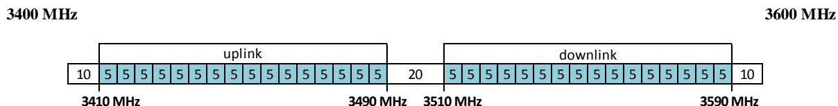
Alternatíva 1: Rozdelenie frekvenčného pásma 3400 – 3600 MHz s FDD
