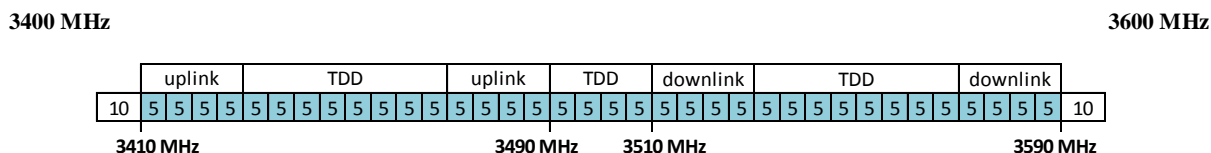
Alternatíva 2: Rozdelenie frekvenčného pásma 3400 – 3600 MHz s TDD (uplink a downlink sú zobrazené z dôsledku existujúceho individuálneho povolenia v danom frekvenčnom úseku)
