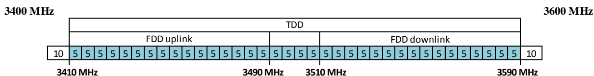
Alternatíva 3: Rozdelenie frekvenčného pásma 3400 – 3600 MHz s kombináciou TDD a FDD
