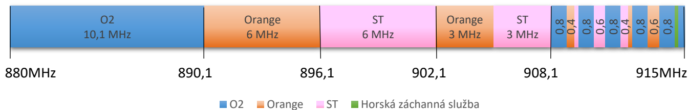
Obrázok 3.2: Rozdeľovanie frekvencií vo frekvenčnom pásme 900 MHz
