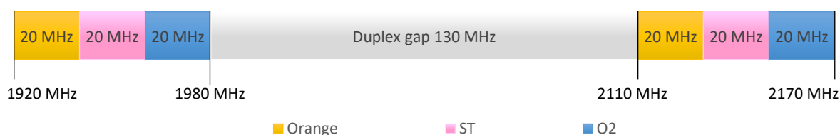
Obrázok 3.3: Rozdelenie frekvencií vo frekvenčnom pásme 2100 MHz
