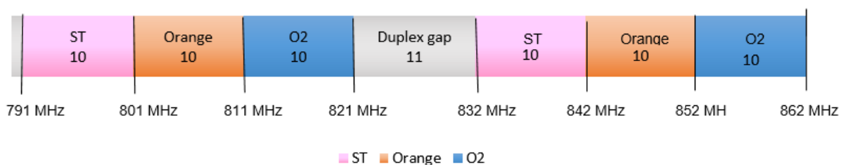
Obrázok 3.1: Rozdelenie frekvencií vo frekvenčnom pásme 800 MHz
