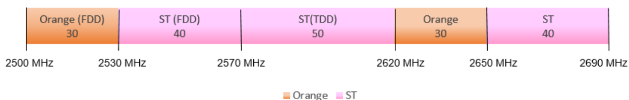
Obrázok 3.4: Rozdeľovanie frekvencií vo frekvenčnom pásme 2600 MHz
