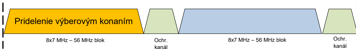
Obrázok 2: Usporiadanie frekvenčného pásma 10 GHz
