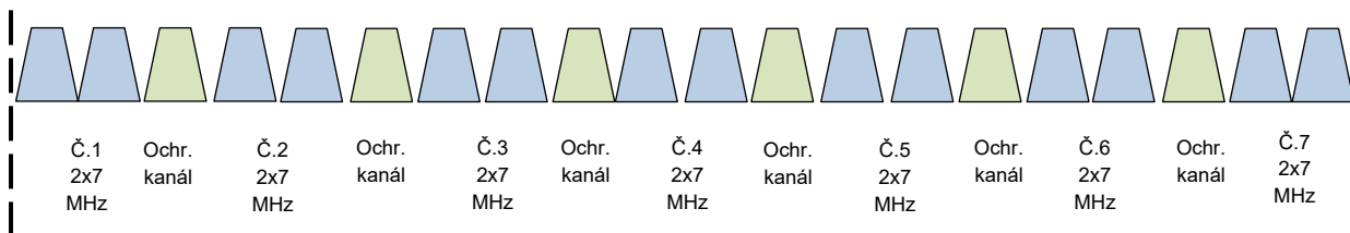
Obrázok 1: Súčasný rozdeľenie frekvenčného pásma 10 GHz
