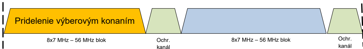
Obrázok 2: Usporiadanie frekvenčného pásma 10 GHz
