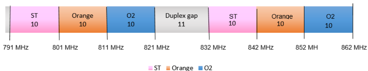
Obrázok 1: Pridelenie frekvencií vo frekvenčnom pásme 800 MHz jednotlivým subjektom
