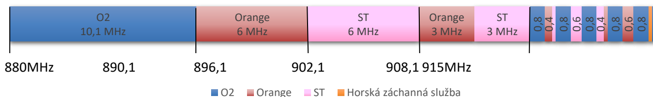
Obrázok 2: Pridelenie frekvencií vo frekvenčnom pásme 900 MHz jednotlivým subjektom
