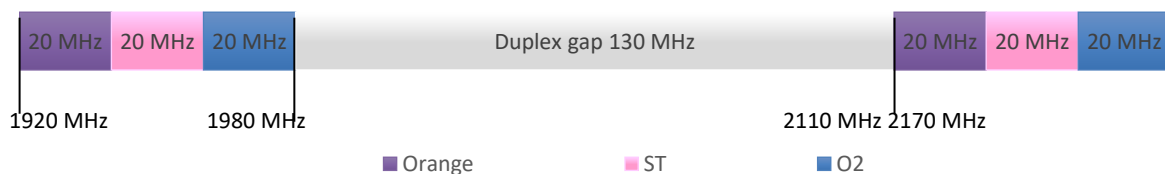
Obrázok 4: Pridelenie frekvencií vo frekvenčnom pásme 2100 MHz jednotlivým subjektom
