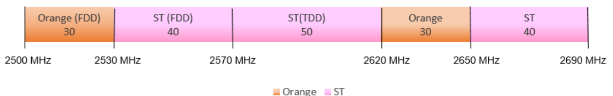
Obrázok 5: Pridelenie frekvencií vo frekvenčnom pásme 2600 MHz jednotlivým subjektom
