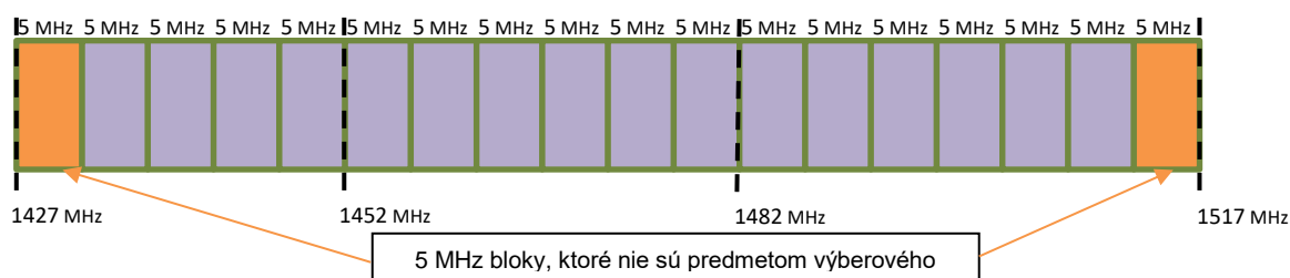
Obrázok 3: Rozloženie frekvenčného pásma 1500 MHz
